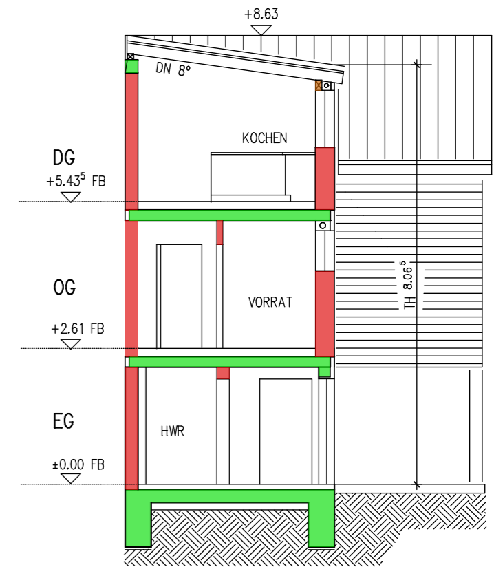
SCHNITT B – B
